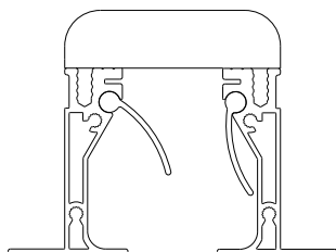
Односторонний горизонтальный выпуск воздуха влево
