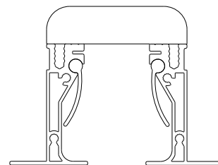
Вертикальный выпуск воздуха
