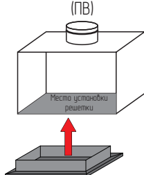
Прямая врезка (ПВ)
