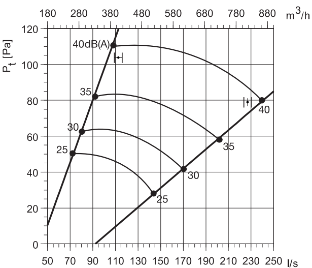
TSO 315+ КСД
