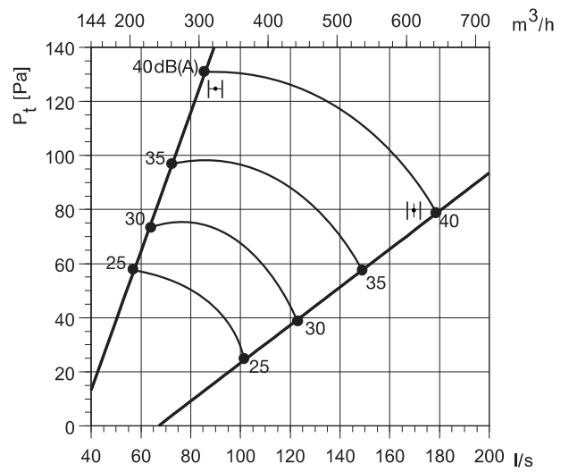
TSO 250+ КСД
