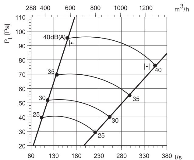
TSO 400+ КСД
