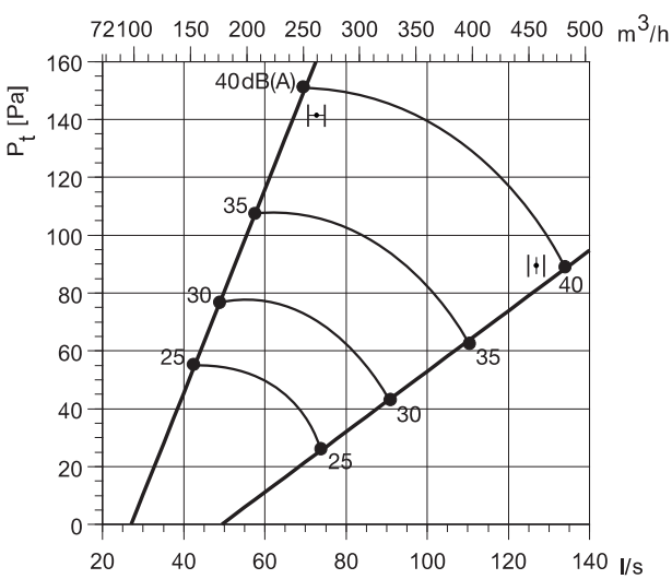
TSO 200+ КСД
