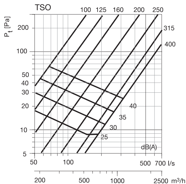
Вытяжной воздух
