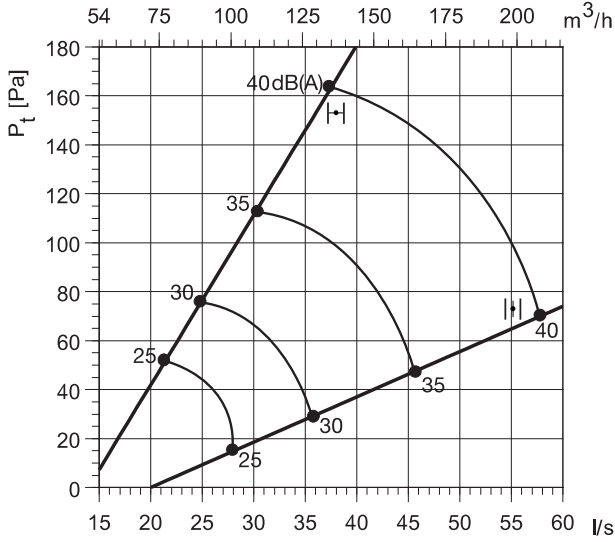
TSO 100-125+ КСД
