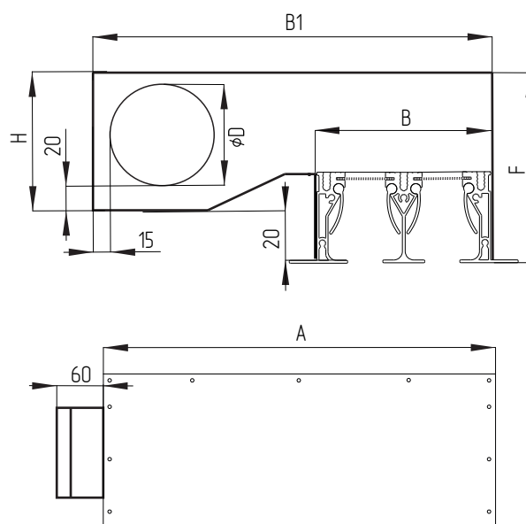
КСД-У торцевой вырезкой
