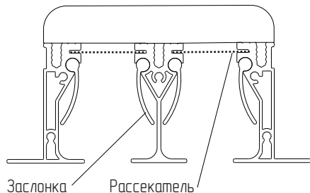
РЭД-TSD-ПФ-3
