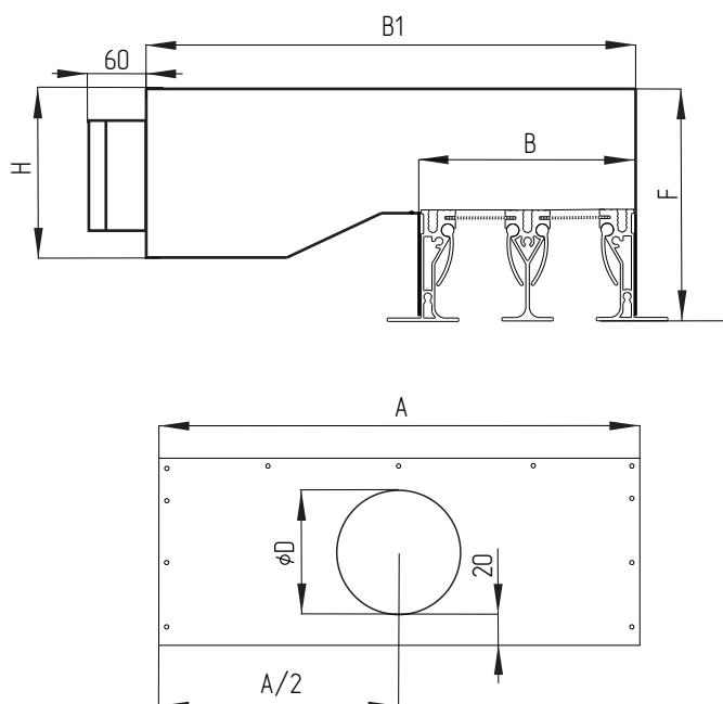
КСД-У с доковой вырезкой
