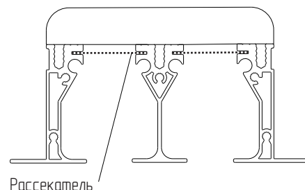
РЭД-TSD-ПФ
