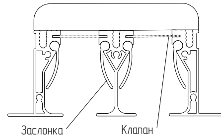
РЭД-TSD-K-3
