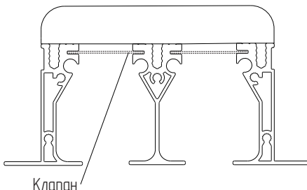
РЭД-TSD-K
