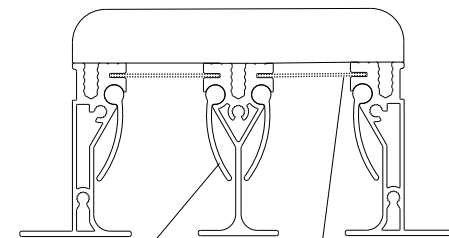
Заслонка
